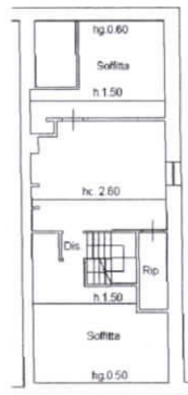
PIANO SECONDO
