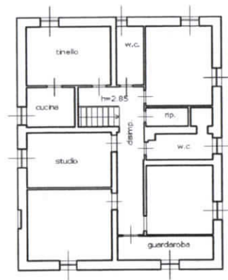
Piano Primo
